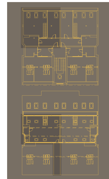
Půdorys podlaží
